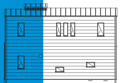
北側立面図
