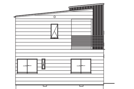
西側立面図
