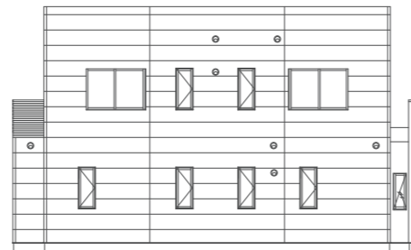
北側立面図
