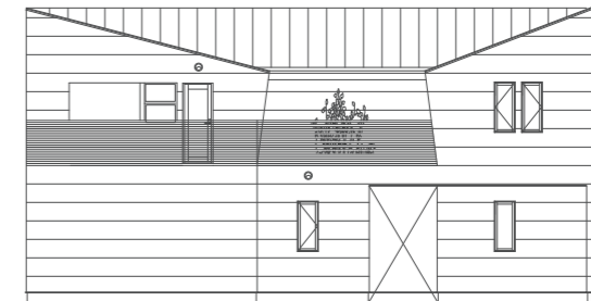
東側立面図
