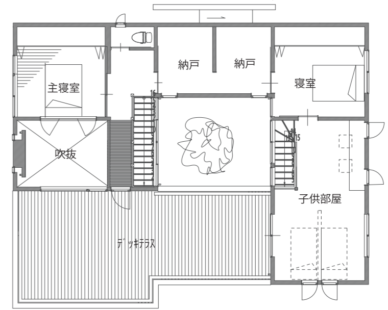
2階平面図
