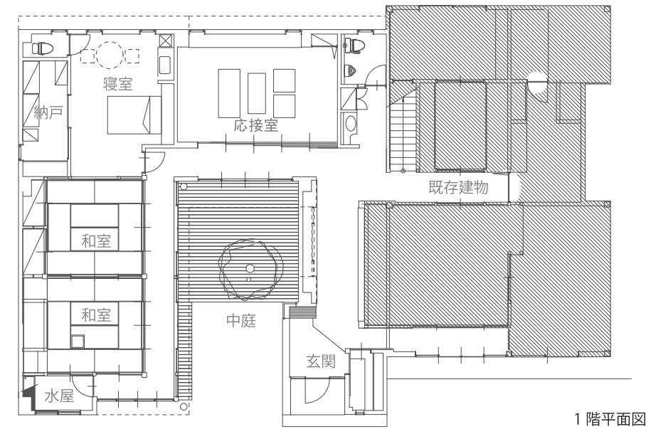
1階平面図
